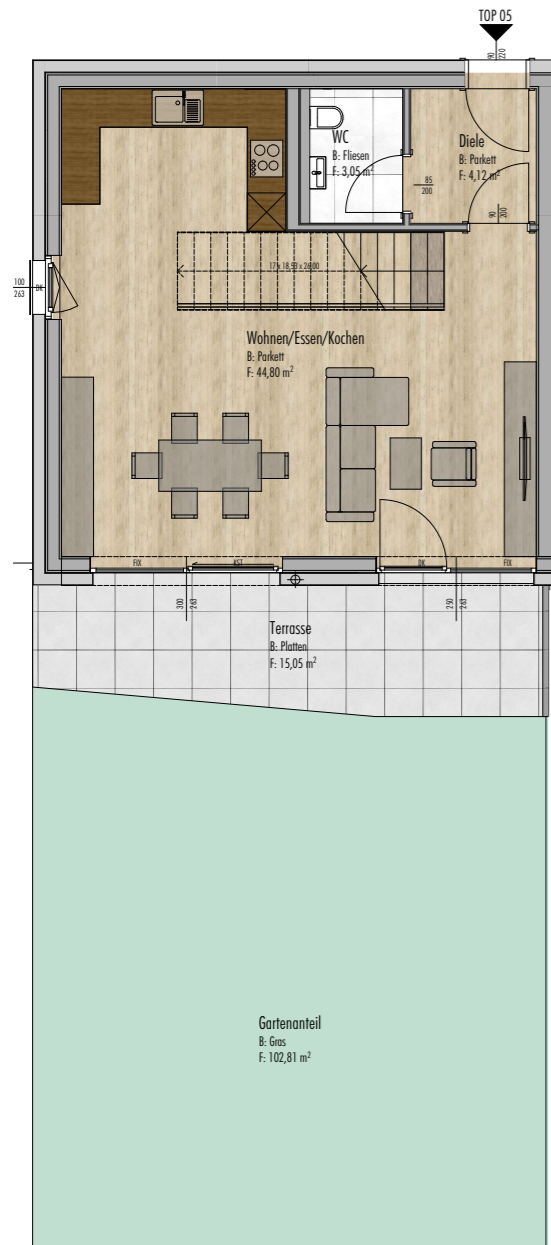
Ebene 0
