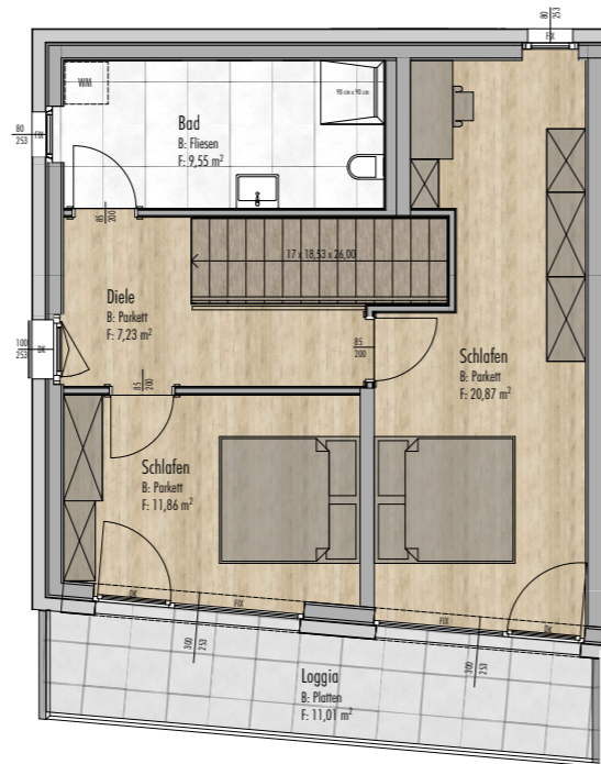
Ebene 1
