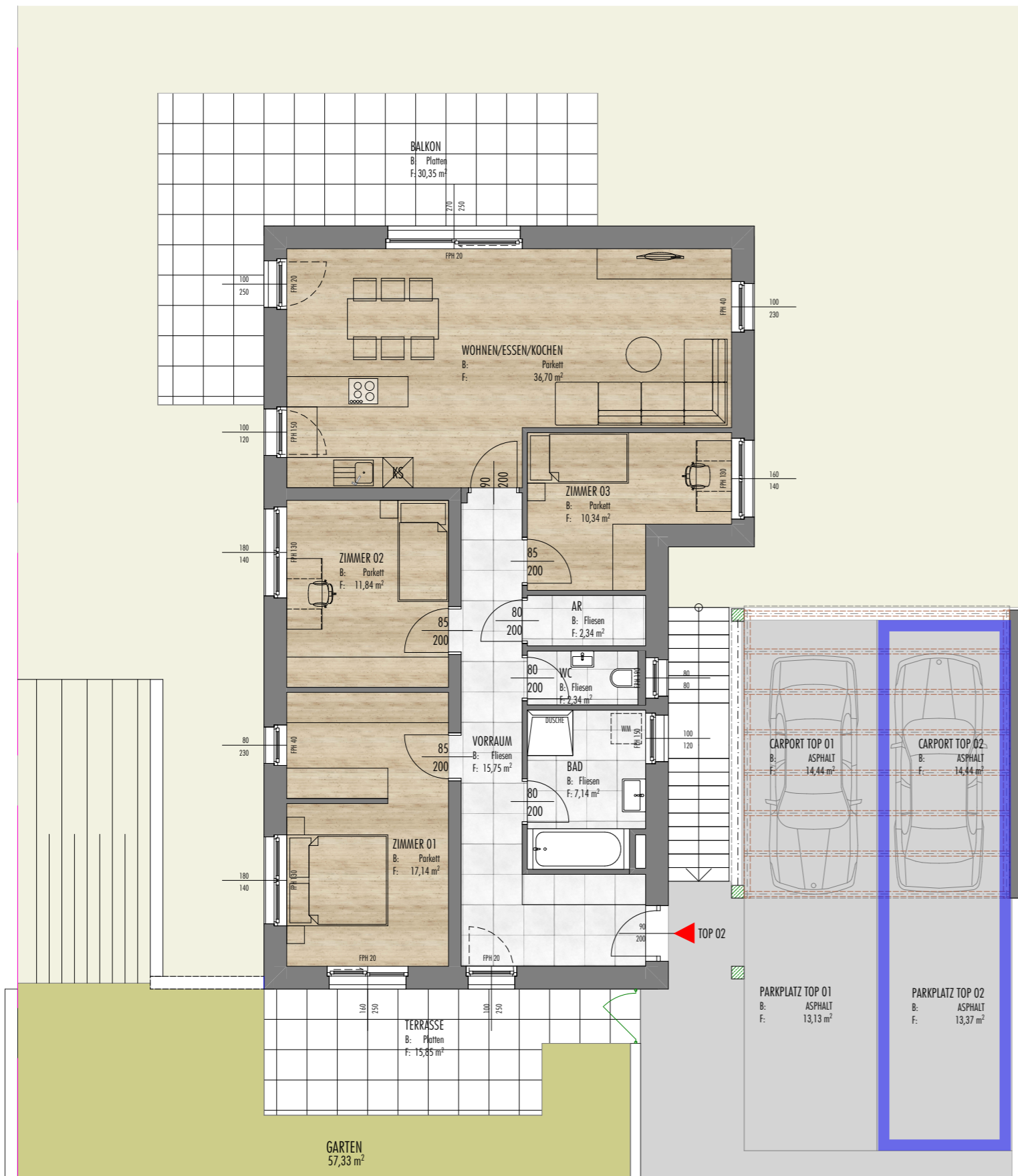
0. Erdgeschoss 1:100
