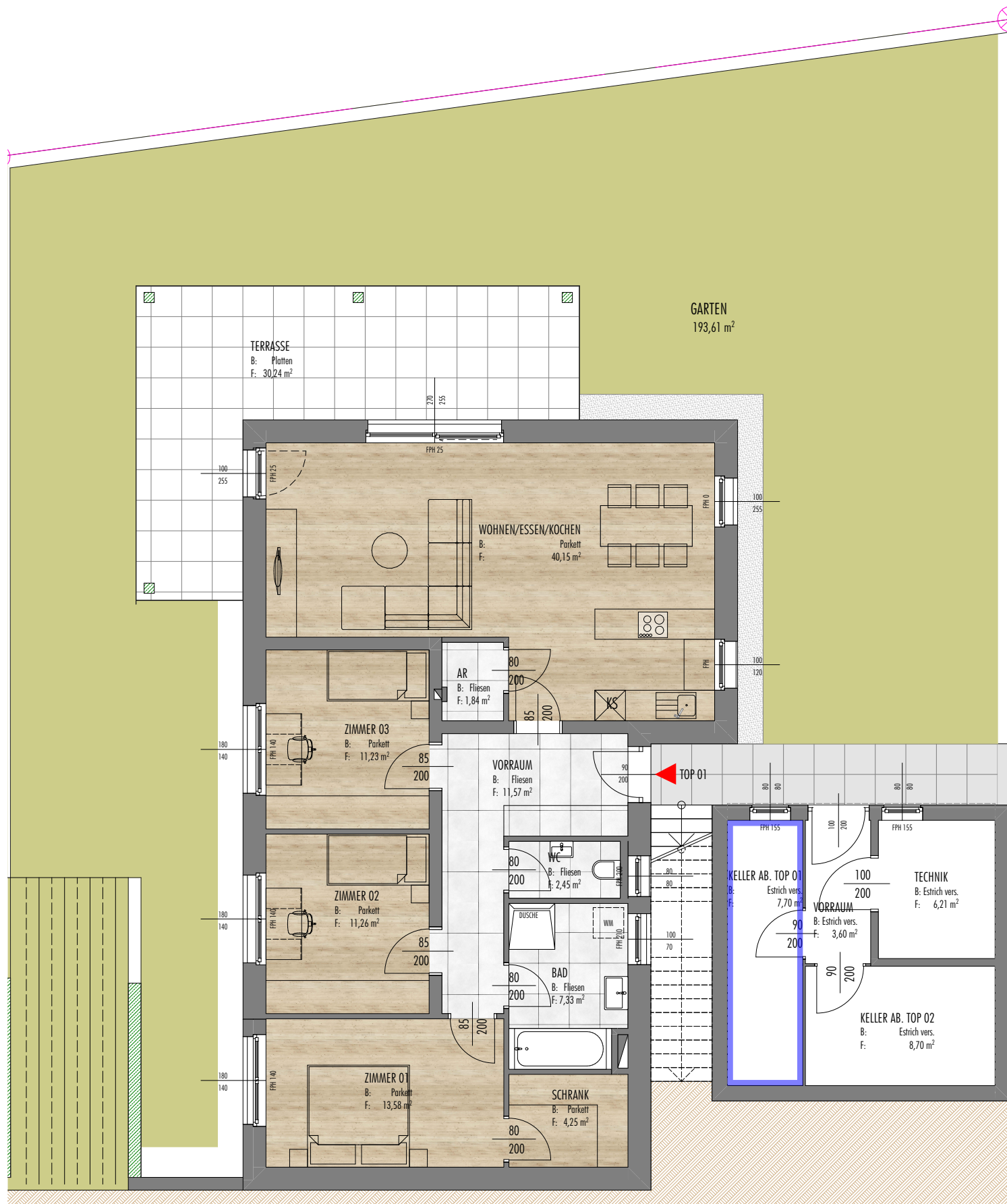
-1. Untergeschoss 1:100
