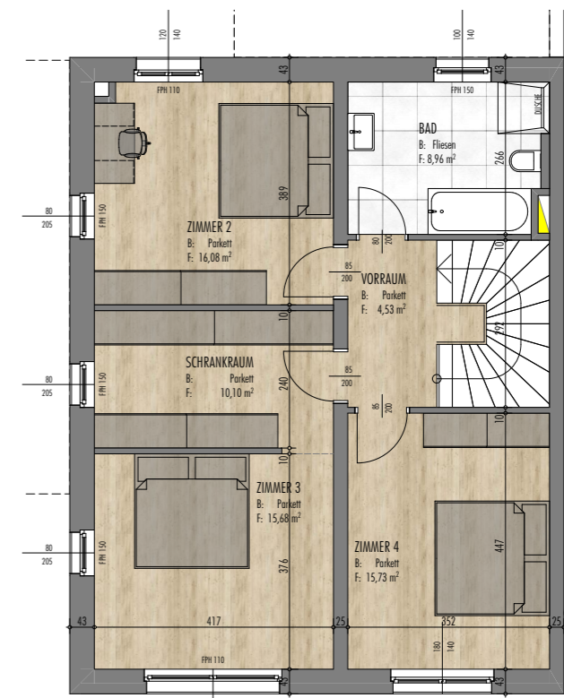
Obergeschoss
