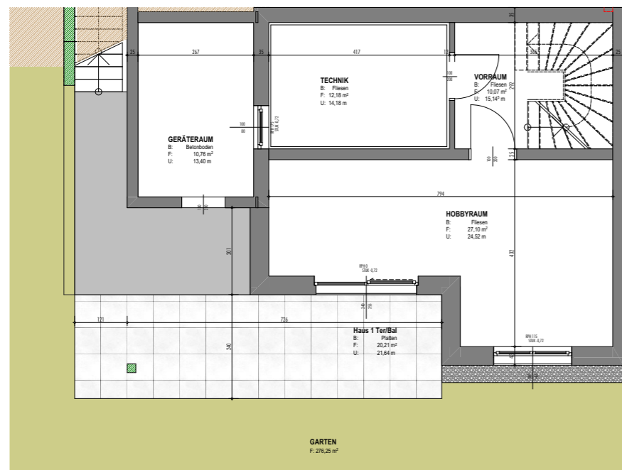
Kellergeschoss
