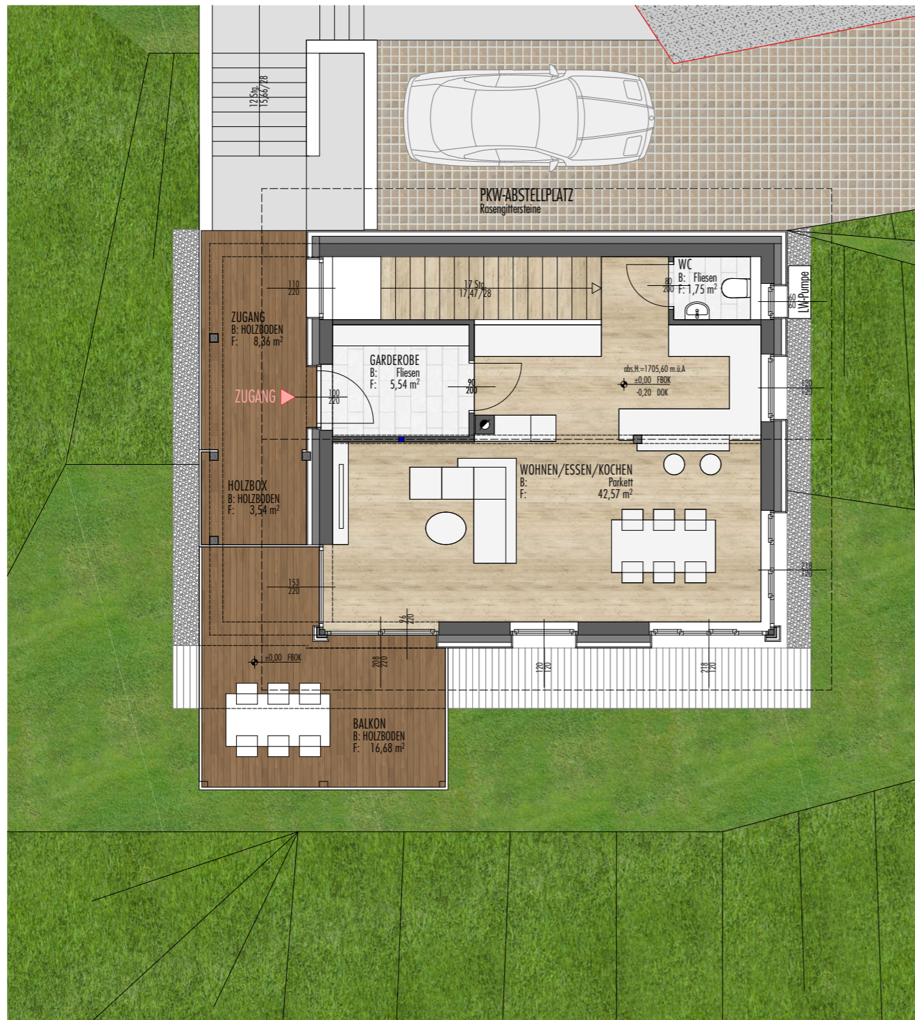
0. Erdgeschoss Haus 3 1:100
