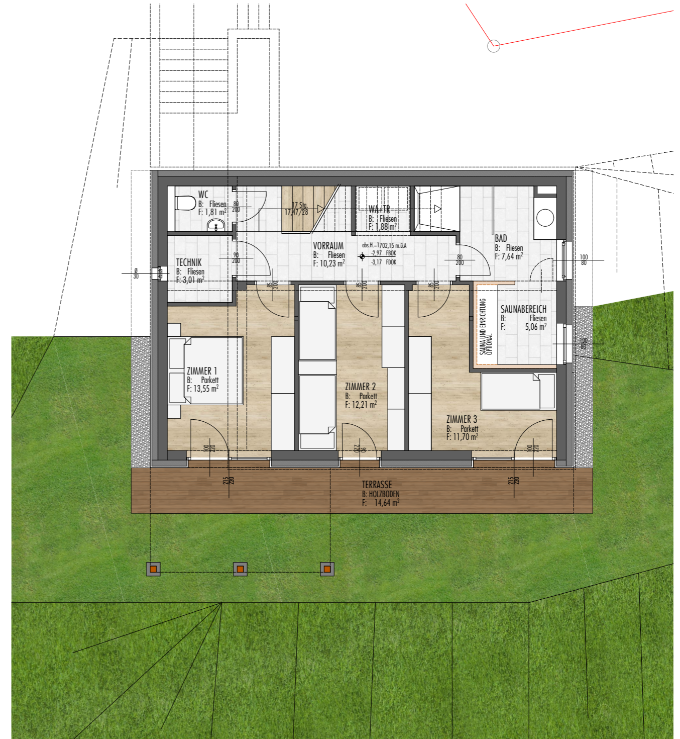
-1. Untergeschoss Haus 3 1:100
