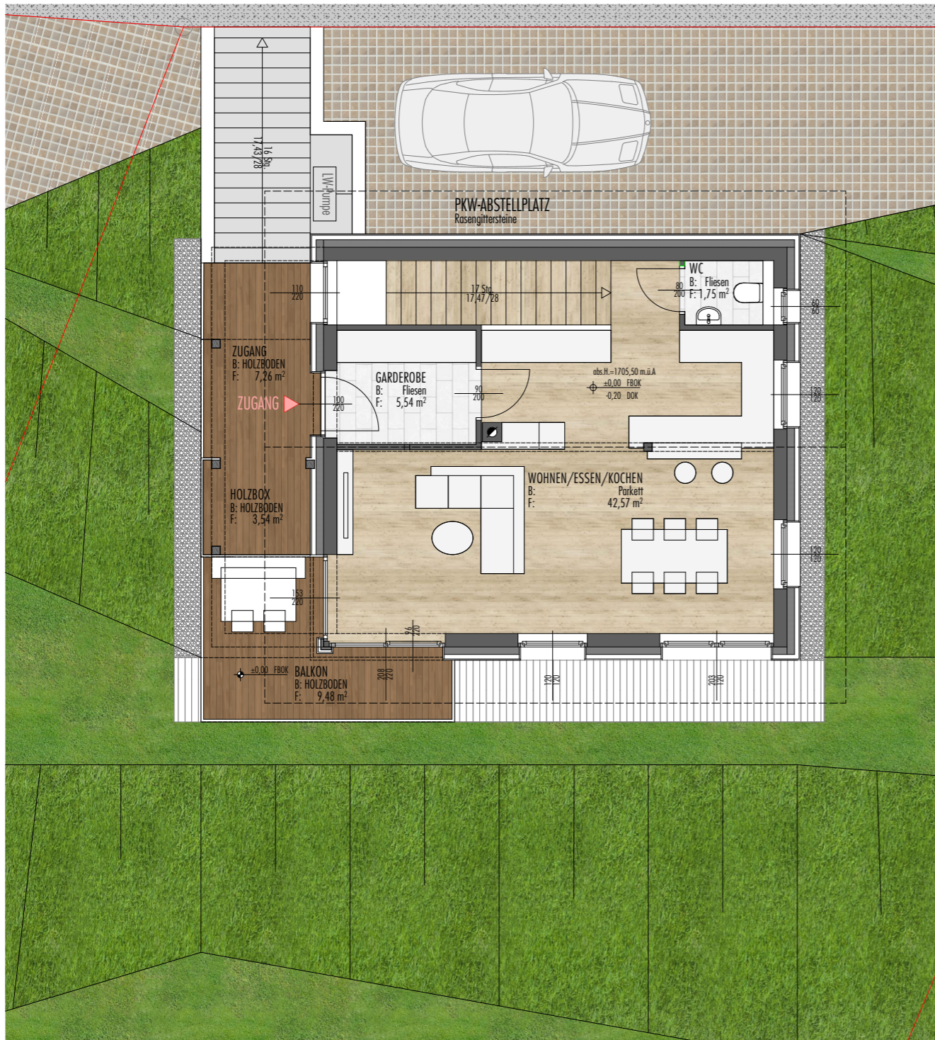
0. Erdgeschoss Haus 2 1:100
