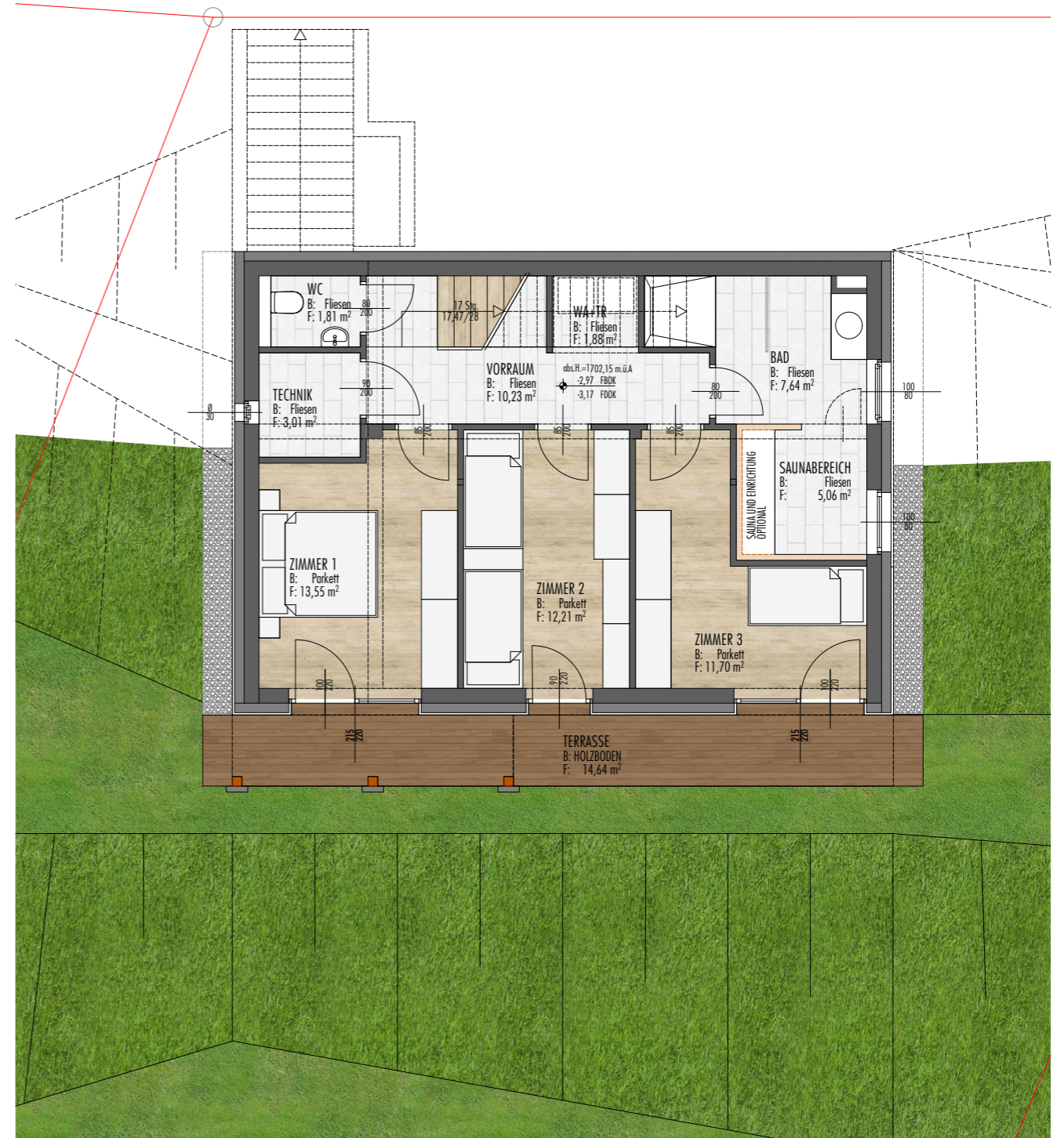
-1. Untergeschoss Haus 2 1:100
