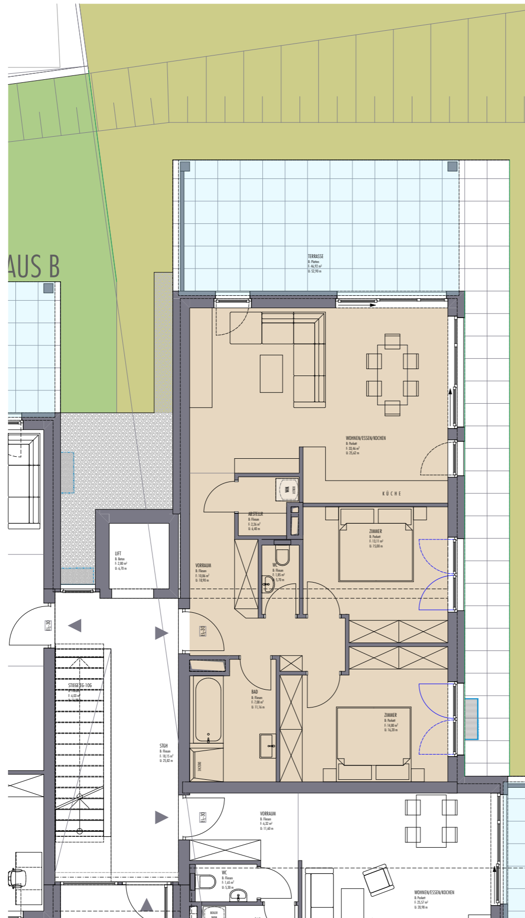
0. Erdgeschoss Haus B 50 1:100
