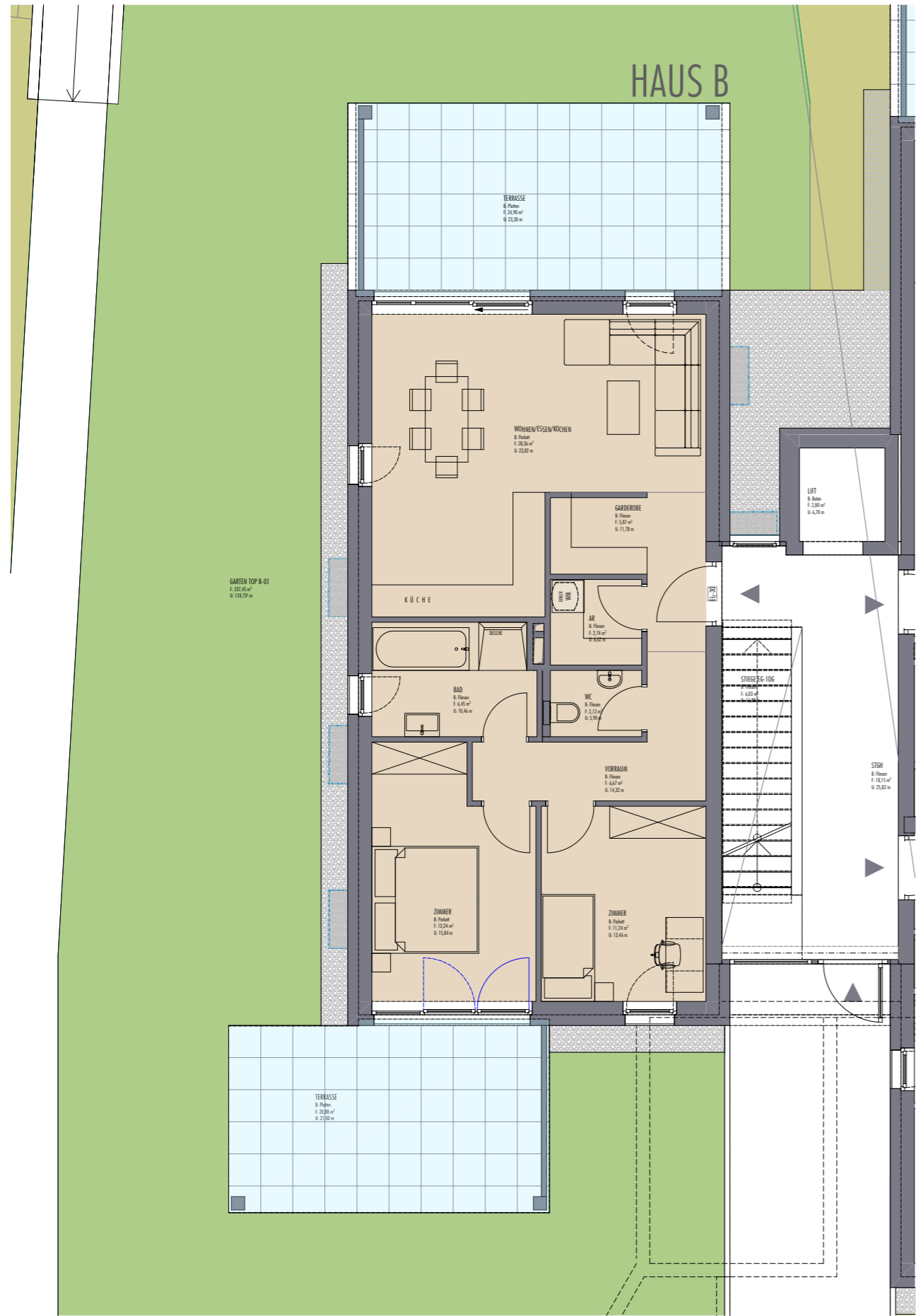
0. Erdgeschoss Haus B 50 1:100
