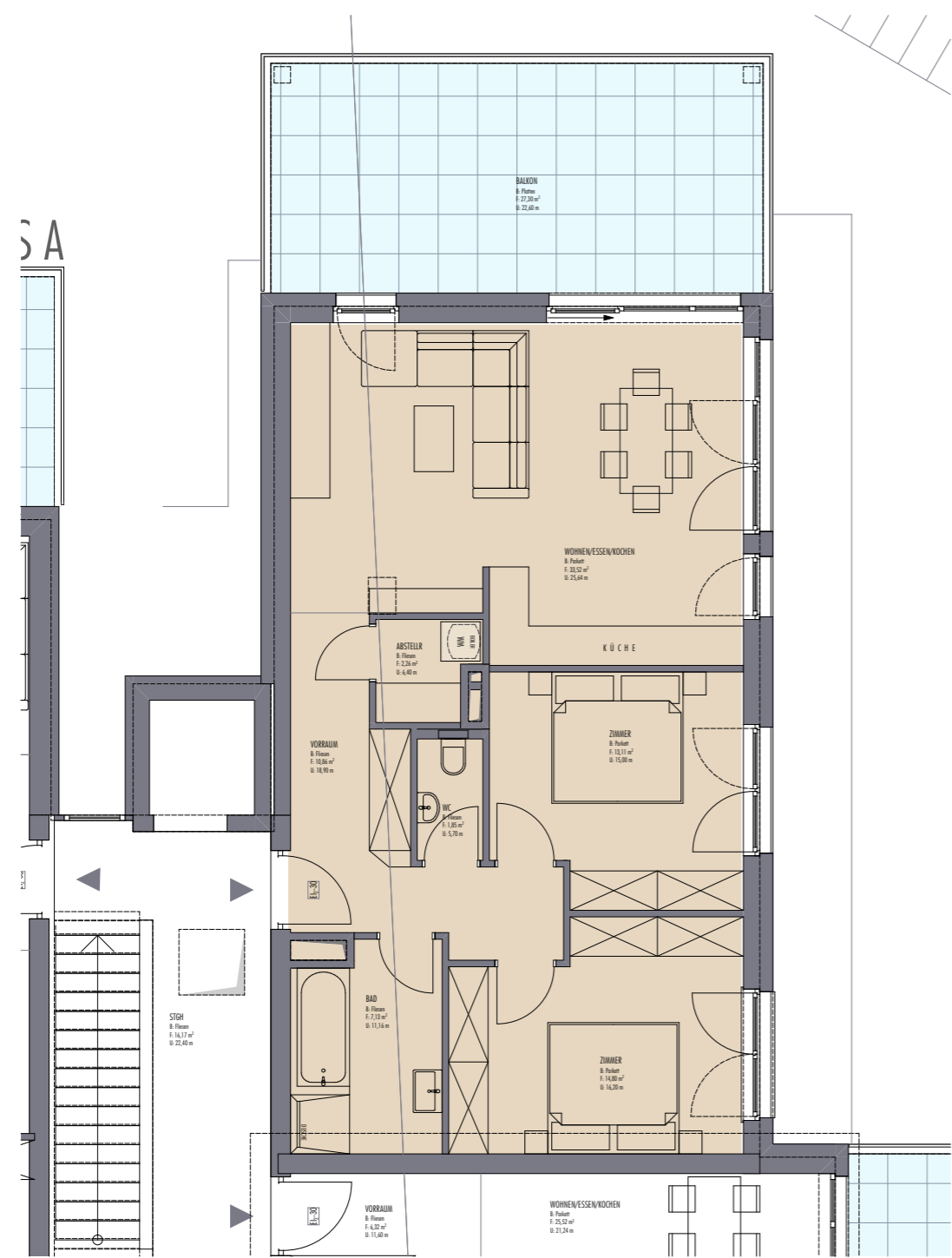
1. Obergeschoss Haus A 50 1:100
