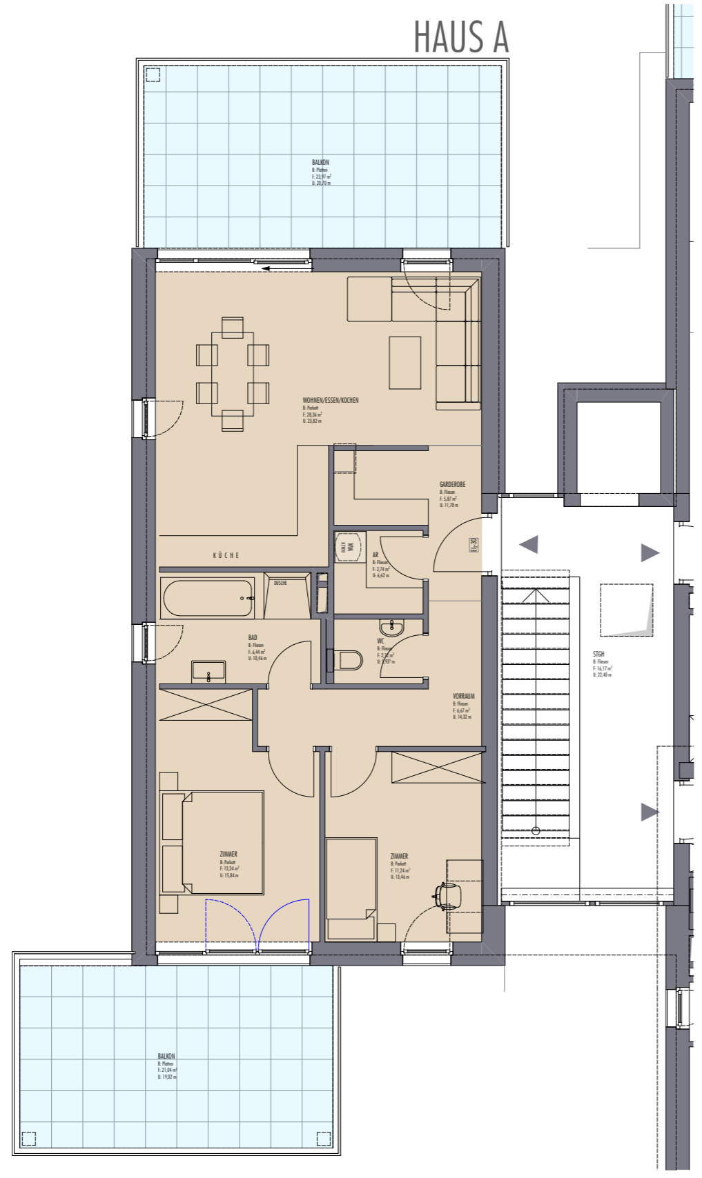
1. Obergeschoss Haus A 50 1:100
