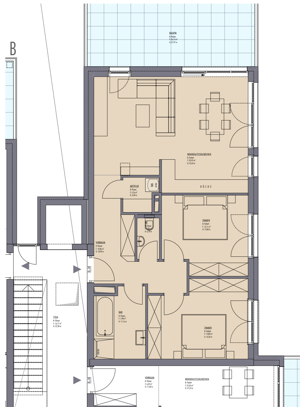
1. Obergeschoss Haus B 50 1:100
